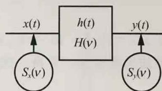
图4.2 线性系统中噪声分析的示意图，上面的符号代表时间行为，下面的符号代表频率行为
